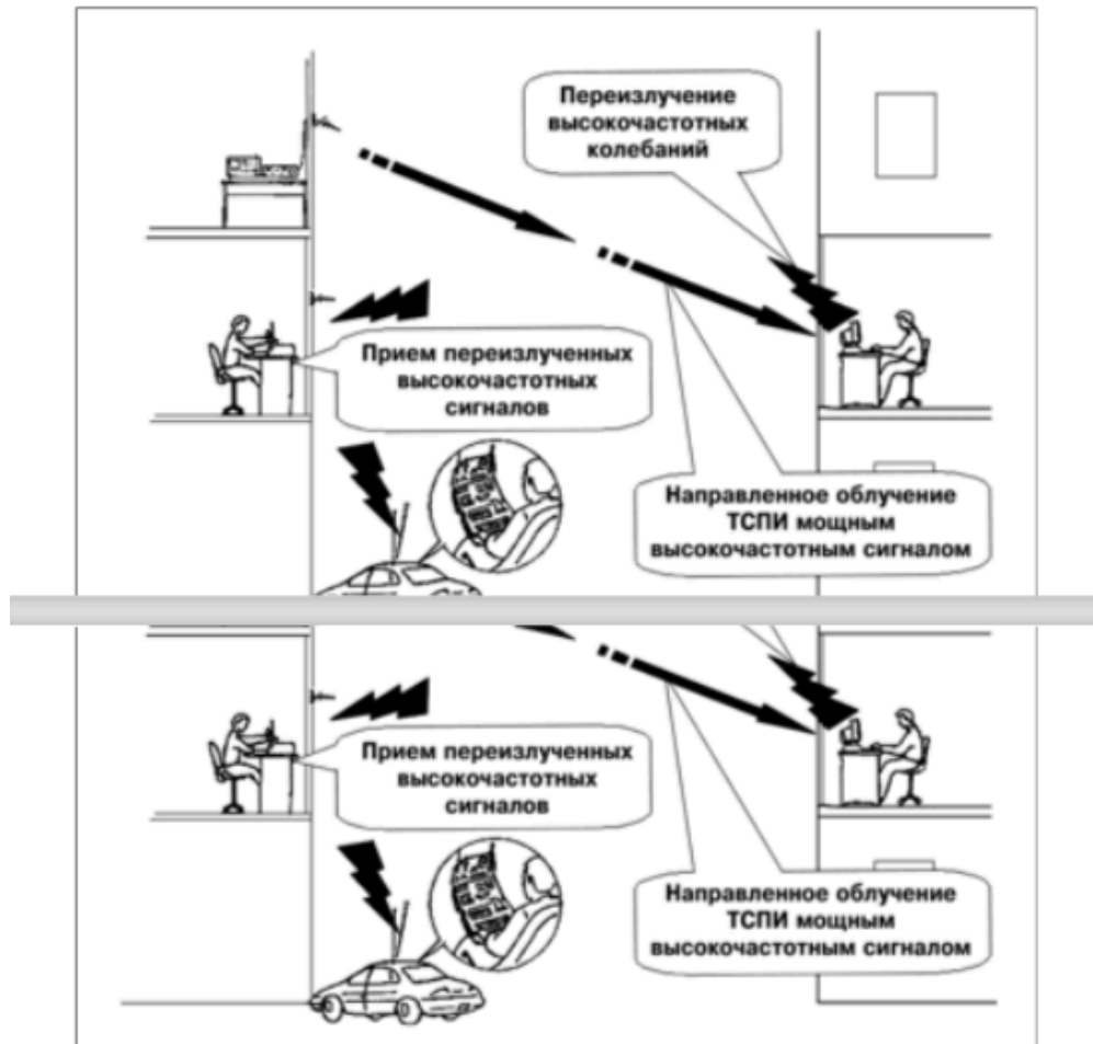
Рис. 3. Перехват информации, обрабатываемой ТСПИ, методом "высокочастотного облучения"
